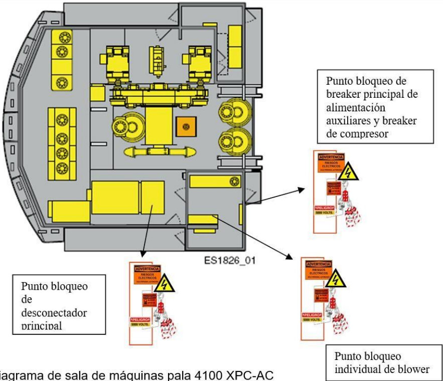
Diagrama de sala de máquinas pala 4100 XPC-AC
