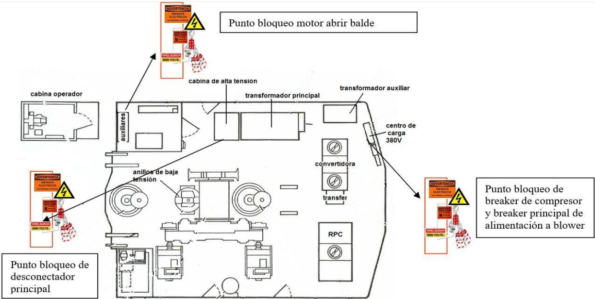
Diagrama de sala máquinas de pala 2800XPB
